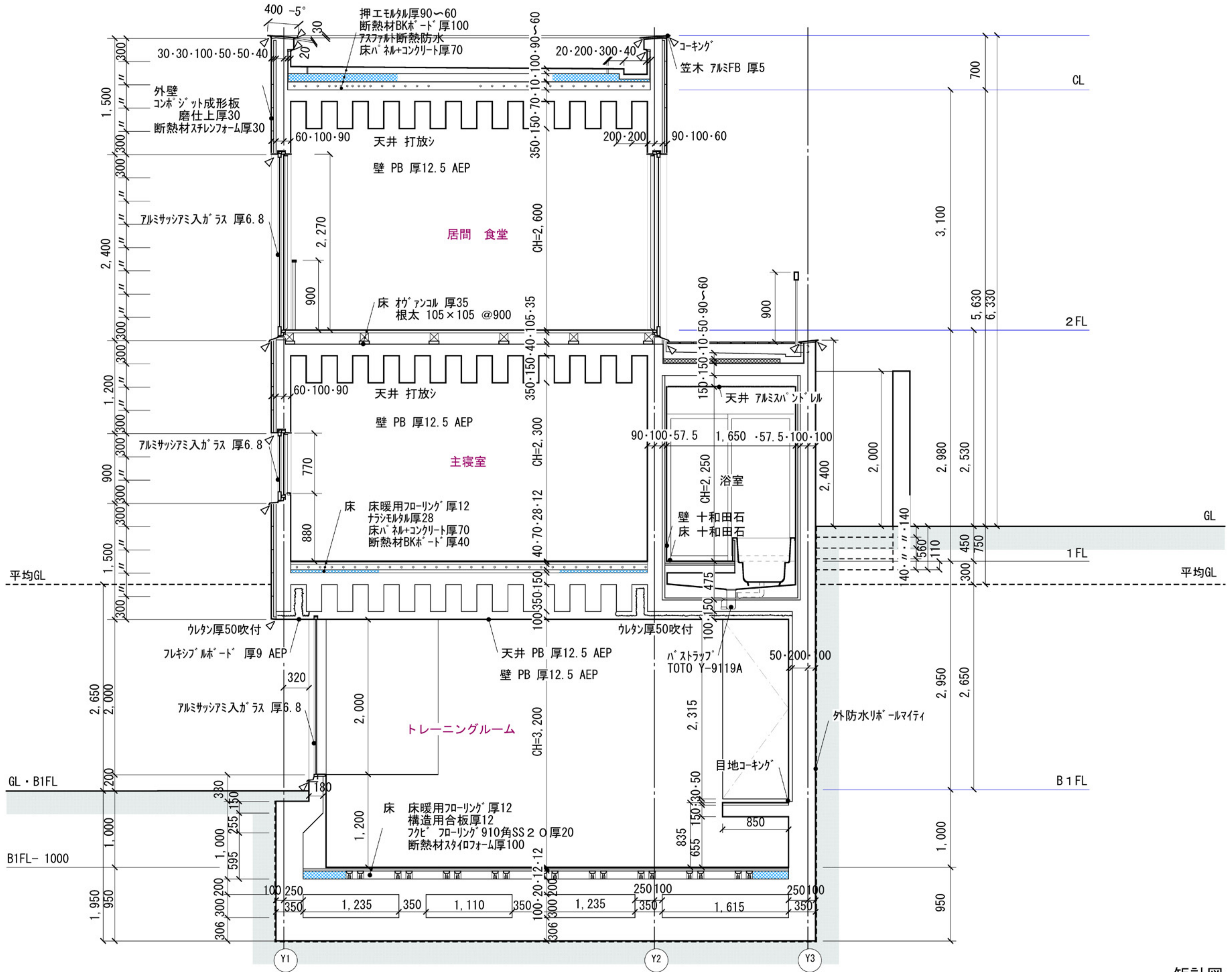
矩計図
